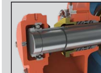
Консистентная смазка подшипника и сальниковое уплотнение
