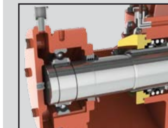
Жидкая смазка подшипника и торцевое уплотнение
